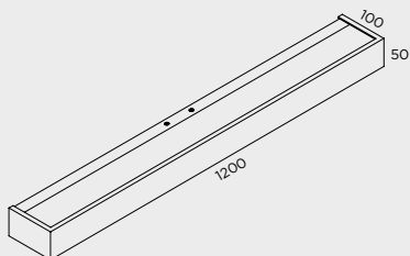
A-811/120 1 x T5 54W IP20
