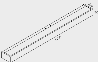
A-811/150 1 x T5 80W IP20
