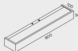
A-811/80 2 x T5 24W IP20
